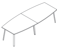
PLF18 2000 / 1100-800 / 740 78.5 kg
