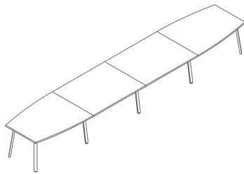
PLF20 5600 / 1100-800 / 740 164.5 kg
