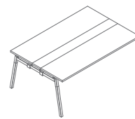
SW28L 1800 / 1210 / 740 67.4 kg
