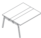
SW24L 1400 / 1210 / 740 53.95 kg
