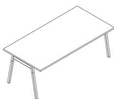
PLD20 2000 / 1000 / 740 57.8 kg
