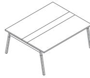
SW46 1600 / 1410 / 740 71.2 kg
