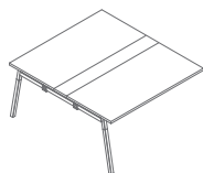
SW33L 1400 / 1610 / 740 64.45 kg
