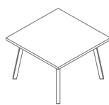
PLD83 800 / 800 / 550 18.7 kg
