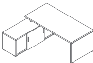
QU19 1900-2164 / 900-1800 / 740 172.55 kg
