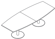
ST15 2800 / 1100-800 / 730 120.1 kg
