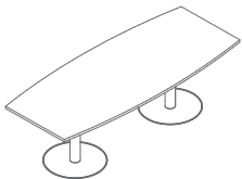
ST24 2400 / 800-1000 / 730 103.75 kg
