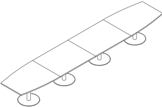
ST17 5600 / 1100-800 / 730 242.3 kg
